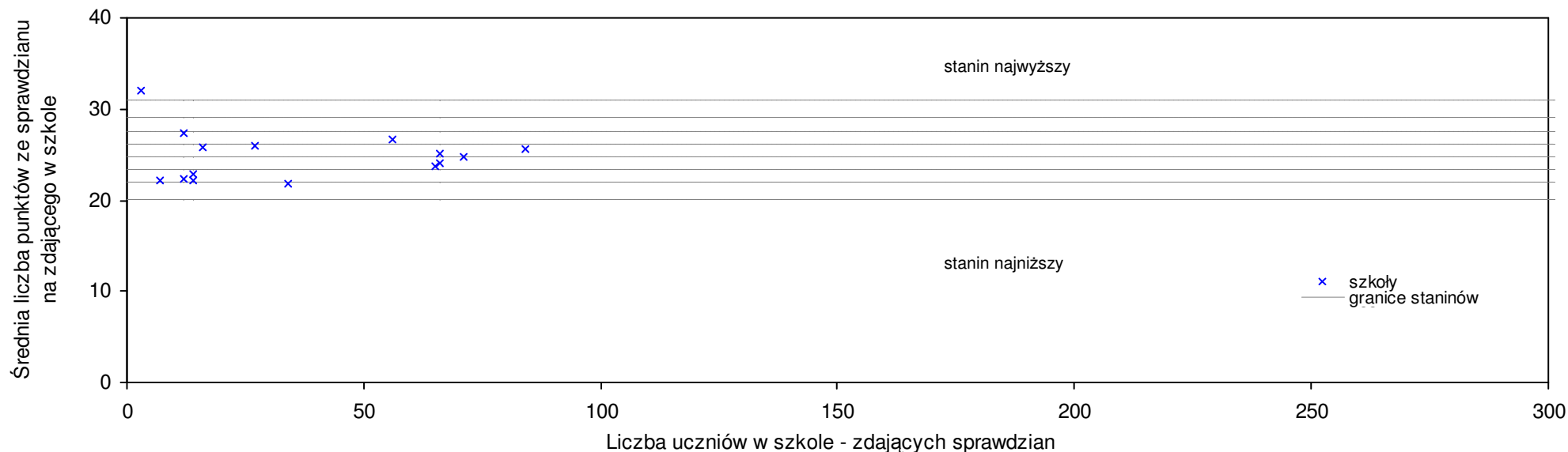
Średnie wyniki szkół na ucznia a liczba zdających sprawdzian w szkole - dla pow. ślubickiego
